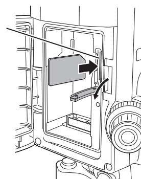
Гнездо SIM-карты
