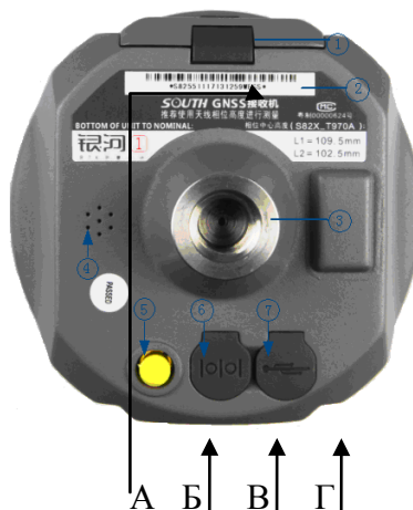
Рисунок 1.2 – Внешний вид приемника со стороны нижней панели
