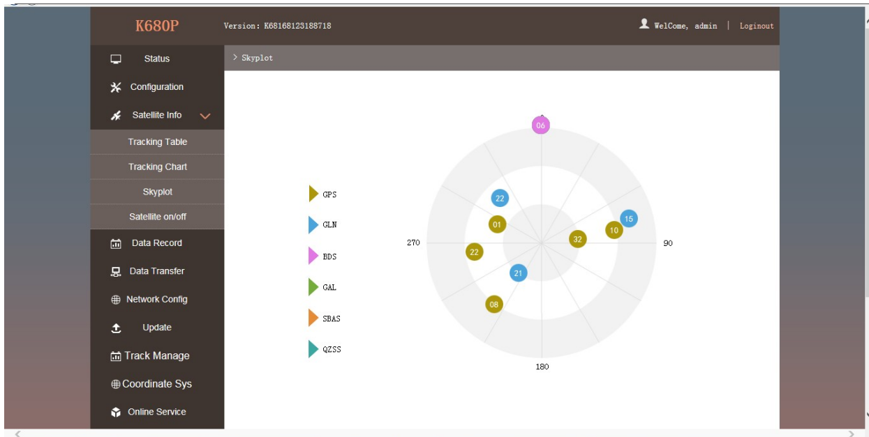
Рисунок 2.3.12 Небосвод
