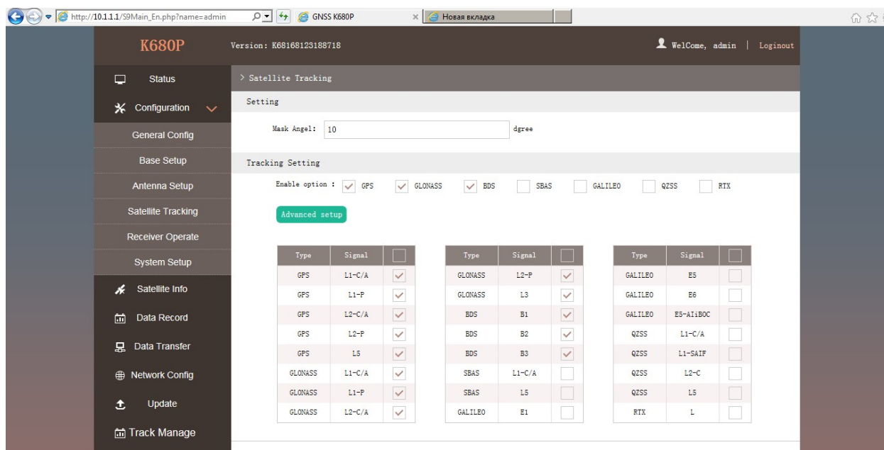
Рисунок 2.3.11 Отслеживание спутников
